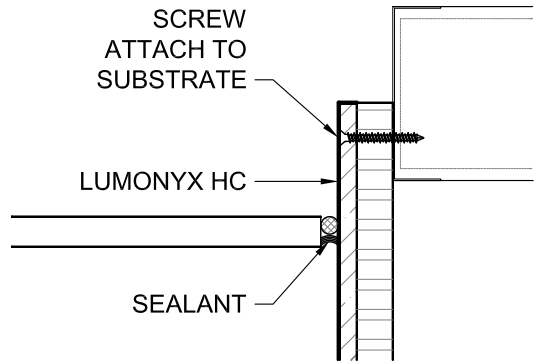
BEAM DETAIL A SCALE: 3" = 1'
